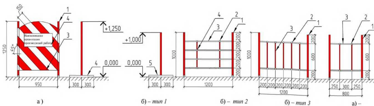
Общий вид ограждения
